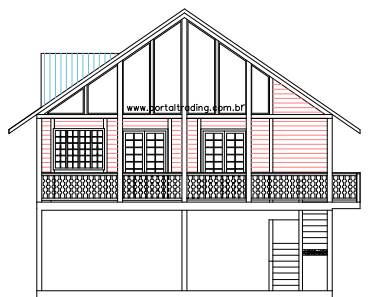
ELEVAÇÃO FRONTAL
