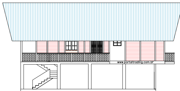
ELEVAÇÃO LATERAL
