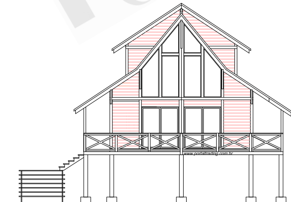
ELEVAÇÃO FRONTAL
